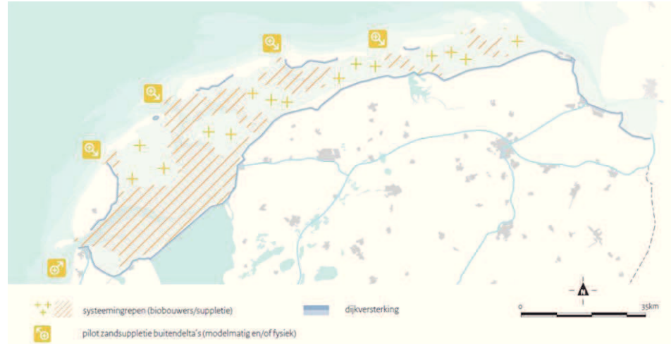
Afbeelding 17 - Systeemingrepen voor buitendelta's en Waddenzee
