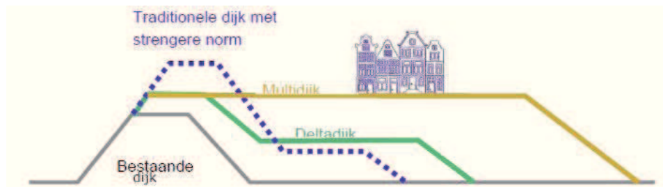
Afbeelding 14 - Kenmerken verschillen en overeenkomsten tussen een Deltadijk en een Multidijk (Van Loon-Steensma et al., 2012a)
