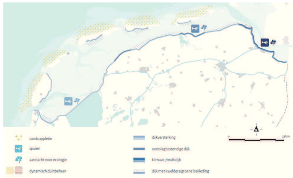
Afbeelding 11 - Optimalisaties voor harde en zachte keringen
