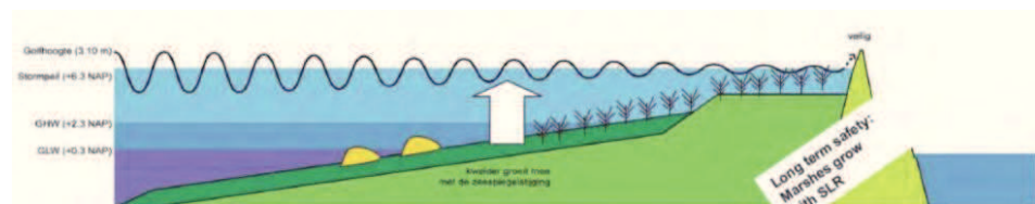
Afbeelding 15 - Principe kwelderwal (Van Loon-Steensma et al., 2012a)
