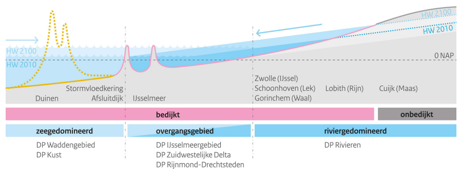
Kaart 2 (figuur) Schematische dwarsdoorsnede van de Nederlandse delta, hoogwatersituatie
