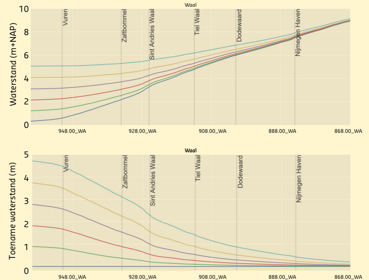
Figuur 5.5 Waterstanden op de Waal bij een gemiddelde Rijnafoer (2200 m 3 /s) en zes verschillende zeewaterstanden bij Hoek van Holland (NAP +0 m tot +5 m). Onder: waterstandsverhoging in vergelijking met de situatie van een zeewaterstand van NAP +0 m.
