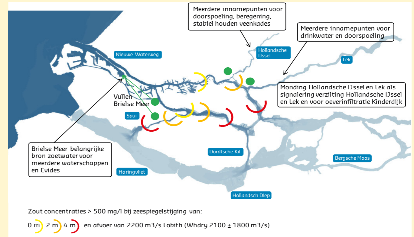
Figuur 6.2 Zoutindringing tijdens vloed voor verschillende zeewaterstanden bij een afvoer van 2200 m 3 /s.
