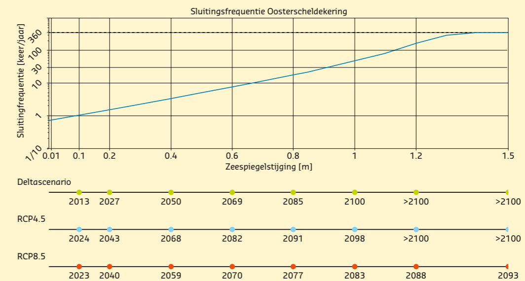
Figuur 5.4 Sluitfrequentie Oosterscheldekering afhankelijk van de zeespiegelstijging. Deze grafiek is bepaald met Hydra-NL. Onder de grafiek is aangegeven wanneer bepaalde niveaus van zeespiegelstijging worden bereikt in de Deltascenario's Warm en Stoom en bij de middenwaarden van de projecties voor extra versnelde zeespiegelstijging. De stippellijn geeft de maximale frequentie aan dat met dit model berekend kan worden. Dit maximum is gelijk aan het aantal getijden per winterhalfjaar (360). Het bereiken van dit maximum impliceert dat in elke getijperiode het sluitcriterium wordt bereikt.
