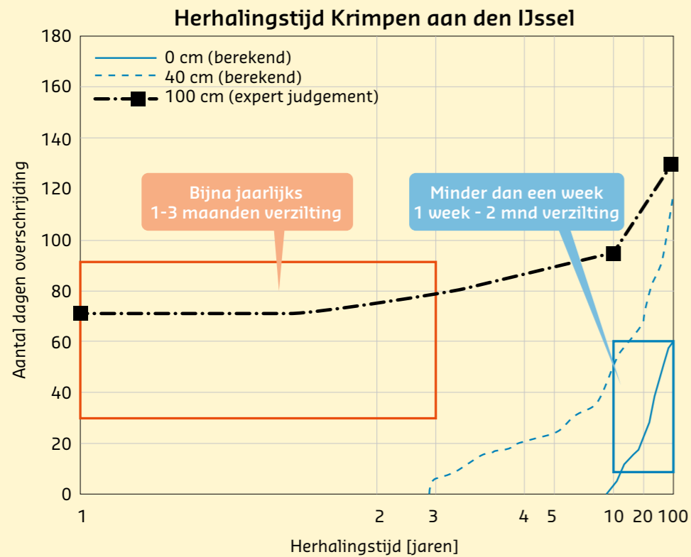
Figuur 6.1 Herhalingstijd van het voorkomen van perioden met langdurige (> 7 dagen) verzilting (>200 mg/l) gedurende het zomerhalffjaar voor verschillende waarden van de zeespiegelstijging (zie legenda). Deze grafieken zijn gebaseerd op een combinatie van simulaties uit het Deltaprogramma en expert judgement.
