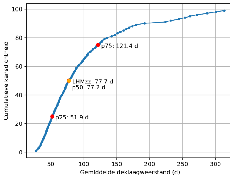
Figuur 3.9 Cumulatieve kansdichtheid van de gemiddelde deklaagweerstand ( d ) in het kwellende gebied in het IJsselmeer, met als rode stippen de 25-, 50- en 75-percentielwaarden weergegeven. De oranje stip is de gemiddelde deklaagweerstand ( d ) in het kwellende gebied in het IJsselmeer zoals die nu is opgenomen in het LHM.
