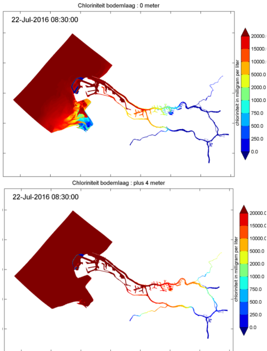
Figuur 2.6 Chlorideconcentratie in Rijn-Maasmond bij zeespiegelstijging (boven: 0 m, onder: 4m) bij een gemiddelde Rijnaivoer van 2000 m 3 /s (Haasnoot et al., 2018).
