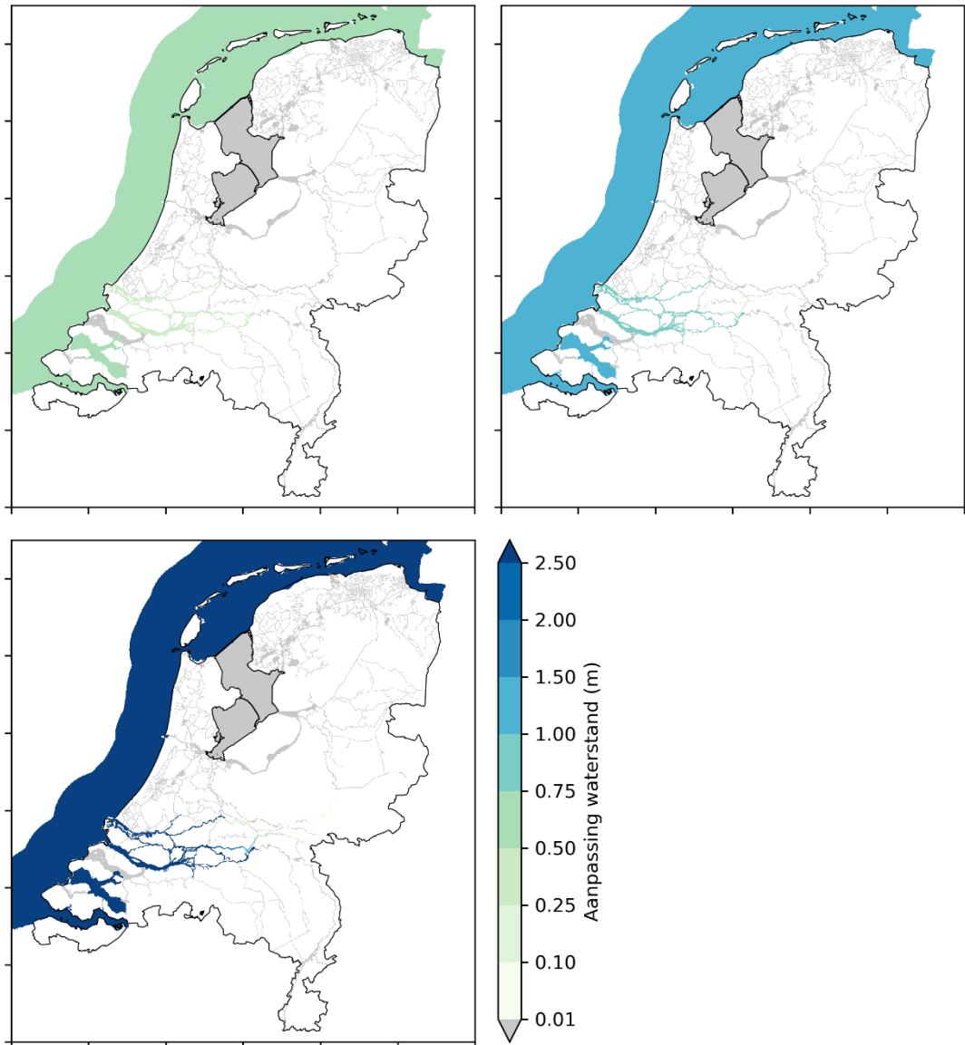
Figuur 3.1 Verschil in opgelegd waterpeil ten opzichte van de huidige situatie in de GHB (zee) en RIV-H (hoofdwatersysteem) randvoorwaarden, voor jaren 2078 (0.5 m ZSS, linksboven), 2129 (1 m ZSS, rechtsboven) en 2277 (3 m ZSS, onder).
