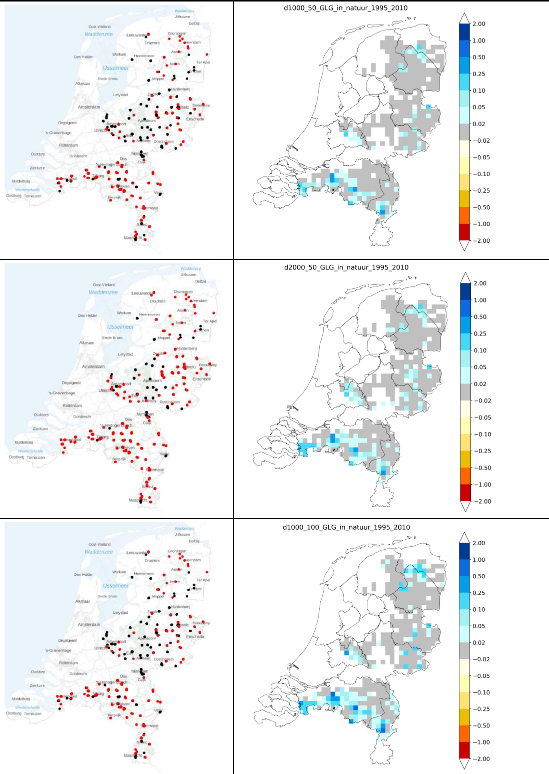
Figuur 3-19 Links: De locaties van de drinkwaterwinningen met in rood de aangepaste winningen. Rechts: De gemiddelde verandering (m) in de GLG voor 1995-2010 ten opzichte van de referentie, gemiddeld over de natuurgebieden in blokken van 6,25 km². Blauwe kleuren tonen een verhoging door de ingevoerde maatregel en geel/rode kleuren een verlaging.
